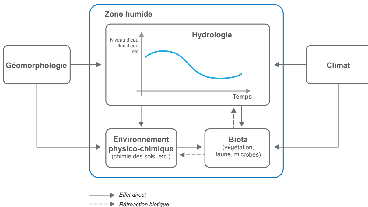
Figure 2. Déterminants du fonctionnement général d'une zone humide (modifié d'après Fustec et Lefevre 2000 issu de NRC 1995).
